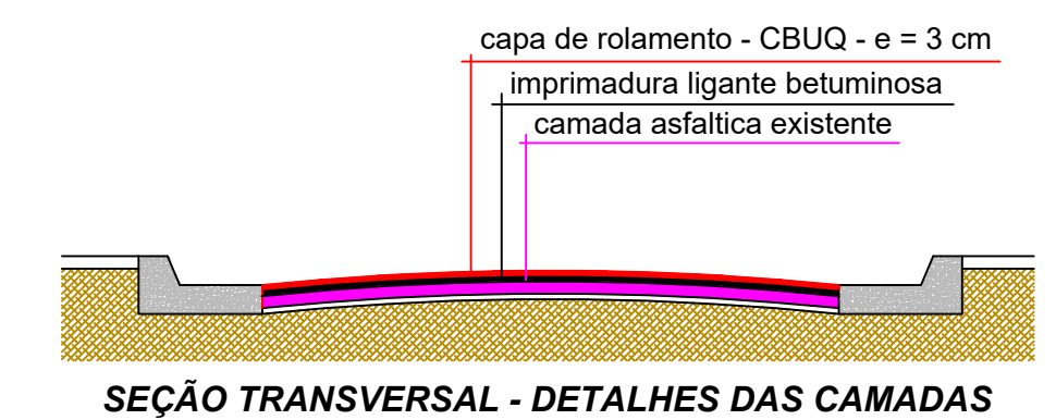
Detalhe 01 - Recapeamento Asfáltico (CBUQ)
