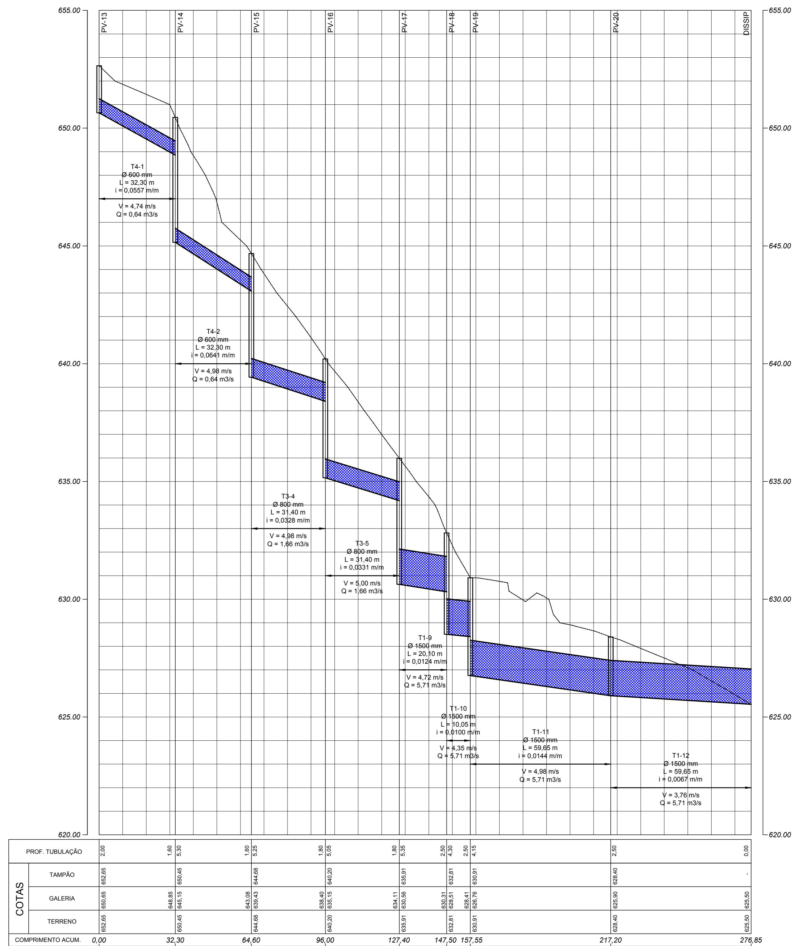
PERFIL REDE DE DRENAGEM - A CONSTRUIR TRECHO 4-1/4-2/3-4/3-5/1-9 A 1-12 ESCALA HORIZONTAL 1:1000 ESCALA VERTICAL 1:100
