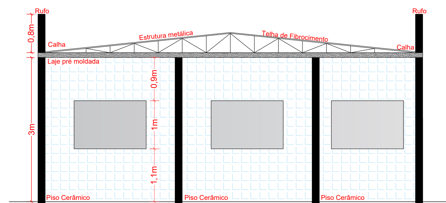
CORTE A.A. ESCALA 1:100
