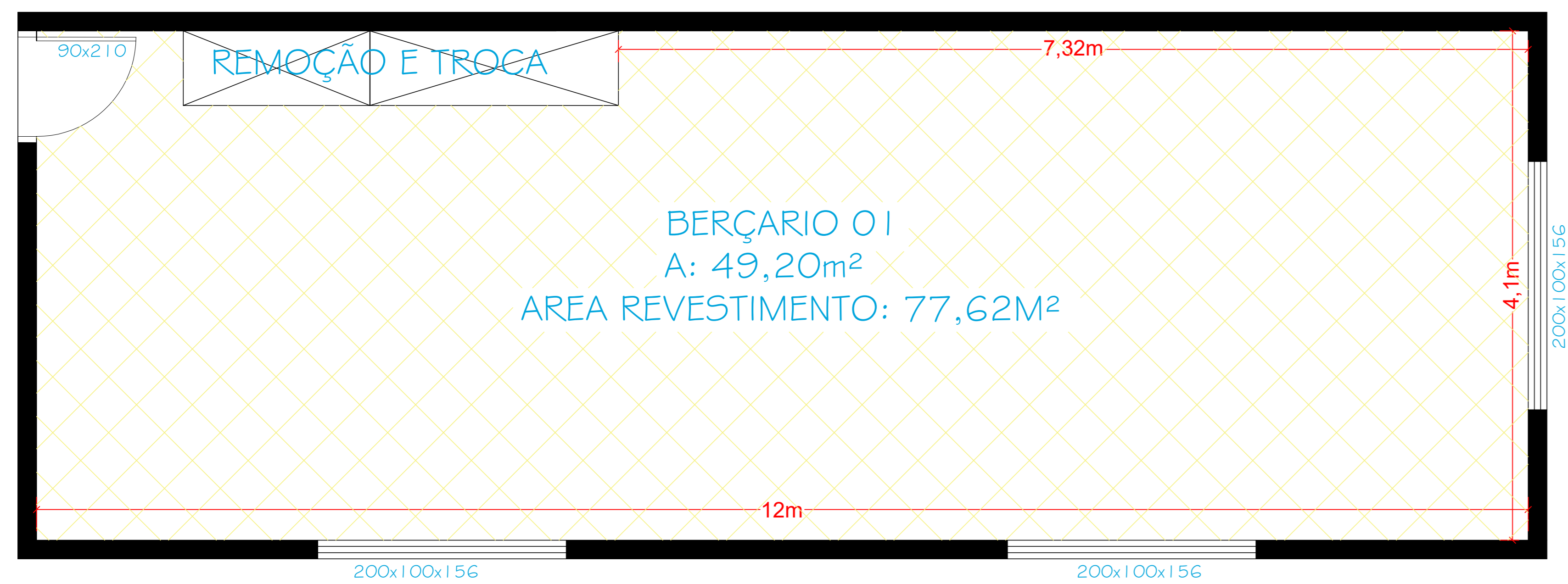
PLANTA BERÇARIO 01 ESCALA 1:100
