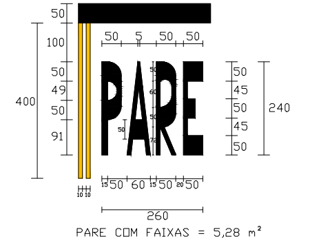
Detalhe 03 - Sinalização Rua Alfredo Raymundo da Silva
