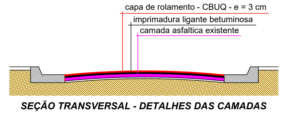
SEÇÃO TRANSVERSAL - DETALHES DAS CAMADAS
