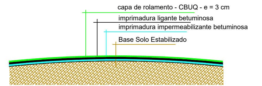
SEÇÃO TRANSVERSAL - DETALHES DAS CAMADAS
